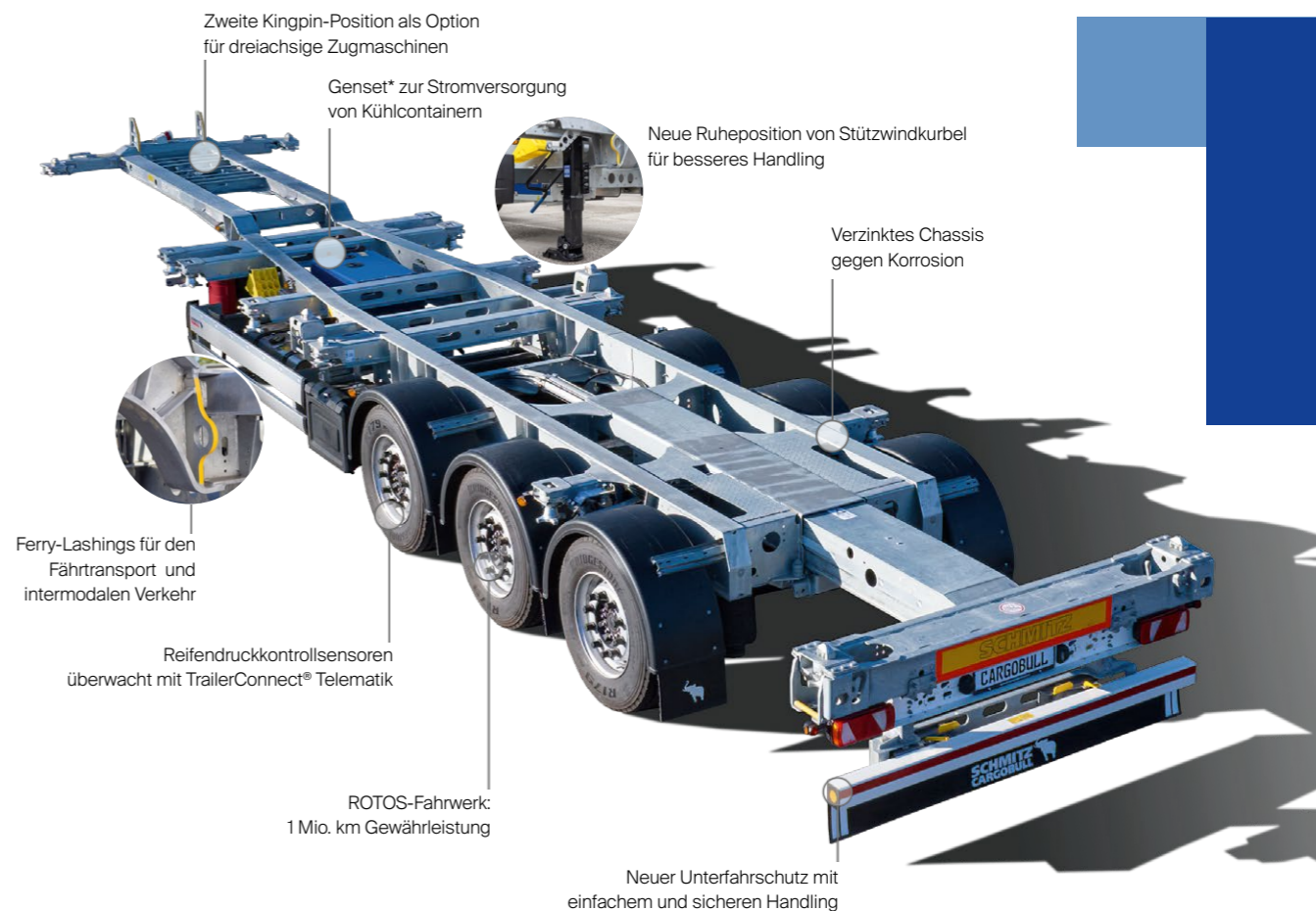
Neu konstruiert: herausfaltbarer Unterfahrerschutz für 45' Container ist einfacher und sicher im Handling ohne lose Teile, die verloren gehen können.
